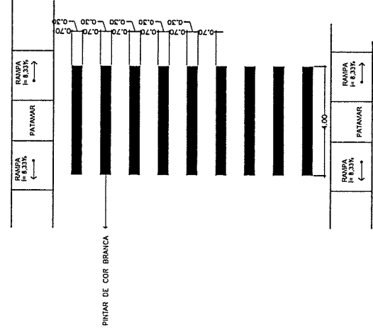
DETALHE DAS FAIXAS DE PEDESTRE SEM ESCALA
